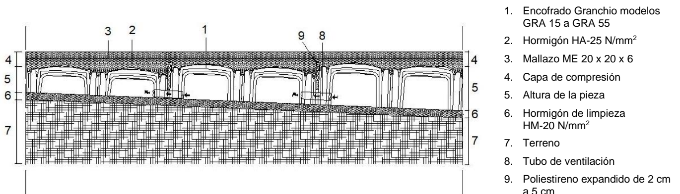
Figura 6.9: Formación de un suelo elevado horizontal a partir de un soporte inclinado.
