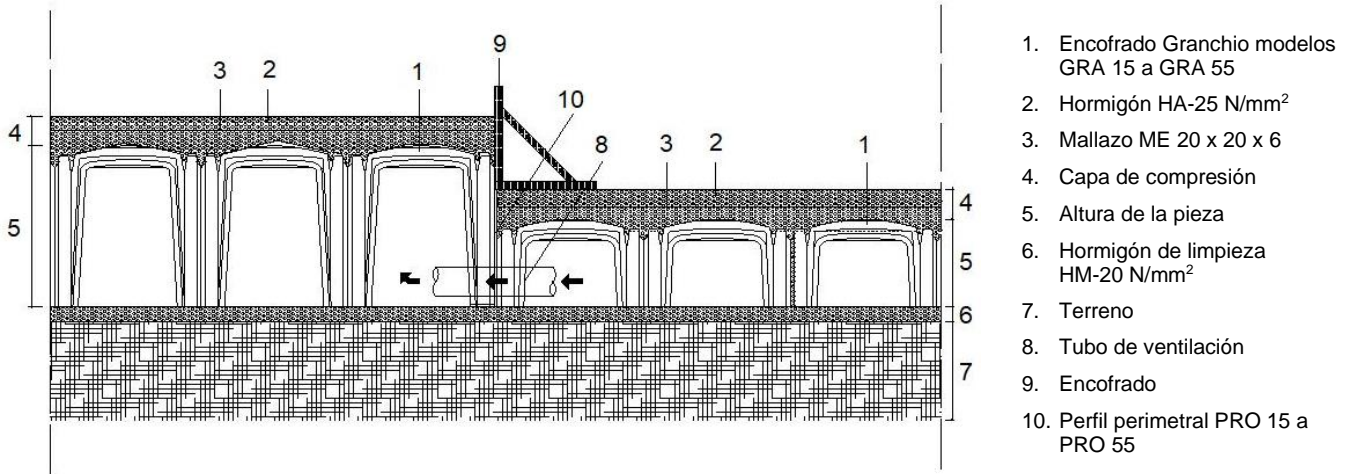
Figura 6.7: Cambio de sección de piezas con encofrado temporal.
