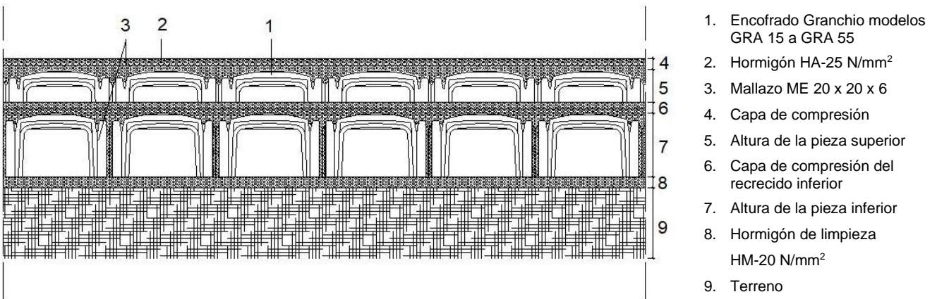
Figura 6.2: Ejecución de recrecio doble con piezas GRA 15 a GRA 55.
