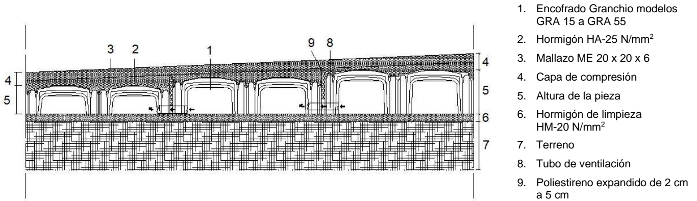
Figura 6.8: Formación de un suelo elevado inclinado a partir de un soporte horizontal.
